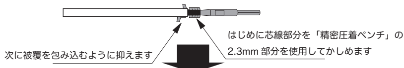
【上面図】
